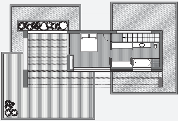
Grundriss OG / 1st floor
