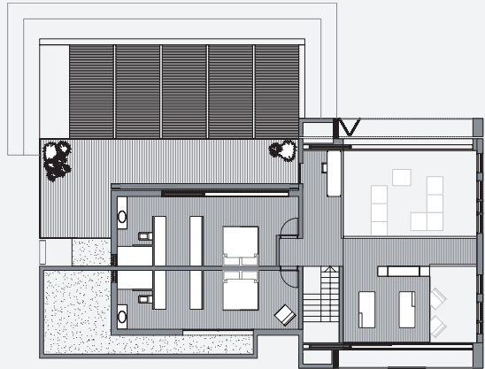
Grundriss OG / 1st floor
